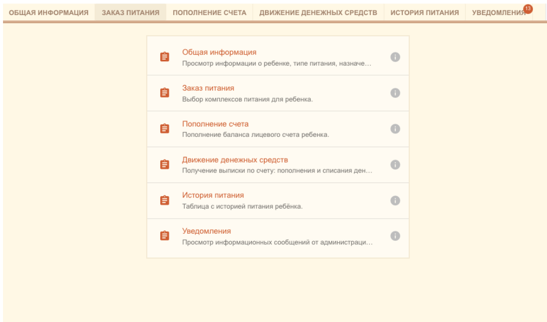
Рисунок 3.3 – Страница УП
